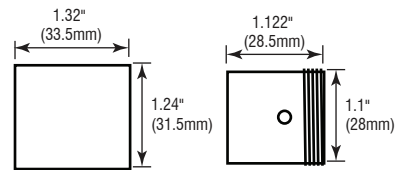
EC—End Cap
